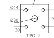
120X120X5 MM PLACA BASE
