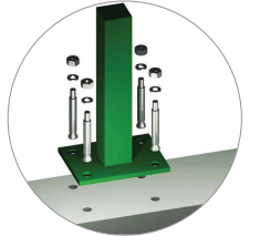
POSTE CON BASE
