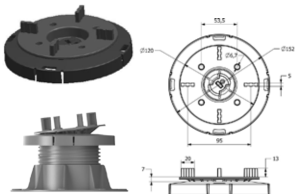
GB-K-RSC Corrector de inclinación hasta 7%
