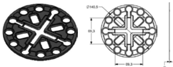
GB-K-S2 Disco de goma estabilizador 2mm
