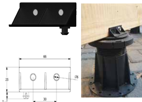
GB-K-AR Accesorio para colocación de baldosas
