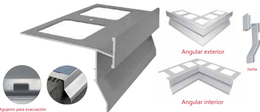
Agujeros para evacuación de agua debajo del azulejo
