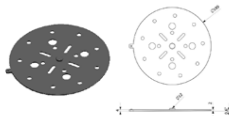
GB-K-SC1 Disco corrector pendiente 1mm
