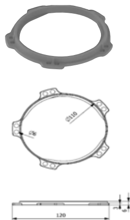
GB-K-L Anillo de fijación para soportes
